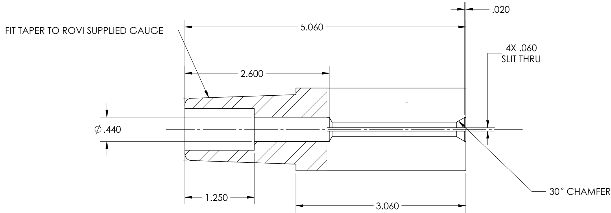
SECTION A-A SCALE 1 : 1
